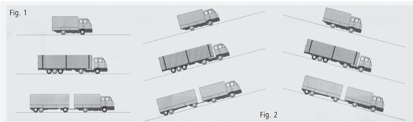
Figura 1: Sugli automezzi da trasporto le catene vanno sempre montate sulle ruote motrici. Sulle motrici e sui semirimorchi le catene vanno montate anche sul penultimo asse. Nei tragitti in salita oppure in discesa, le catene da neve vanno montate come indicato in figura 2 .
